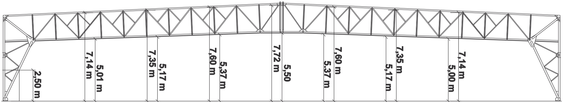
Corte A-A / Pabellón 4
